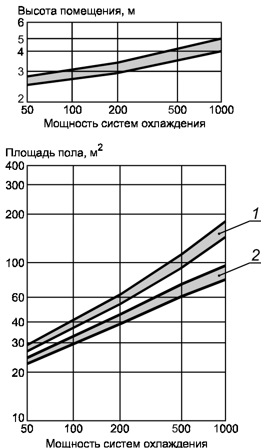
1 — система охлаждения, включая распределение воды; 2 — система повторного охлаждения
