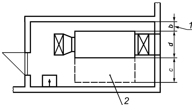
1 — b = 0,4 \times высота оборудования (не менее 0,5 м); 2 — зона обслуживания (ширина зоны обслуживания c должна быть не менее ширины кондиционера d )
