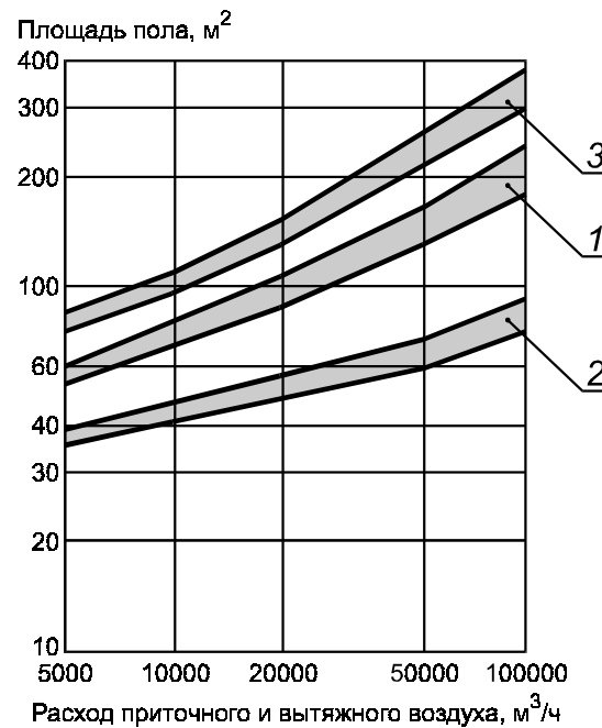
Рисунок А.4 — Высота и площадь вентиляционных камер
